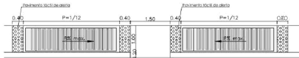
Rampa paralela
