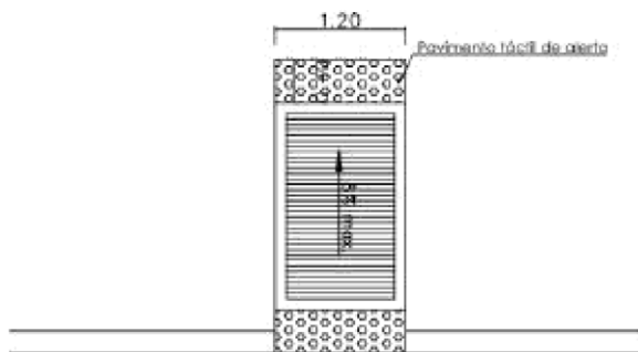
Rampa lineal
